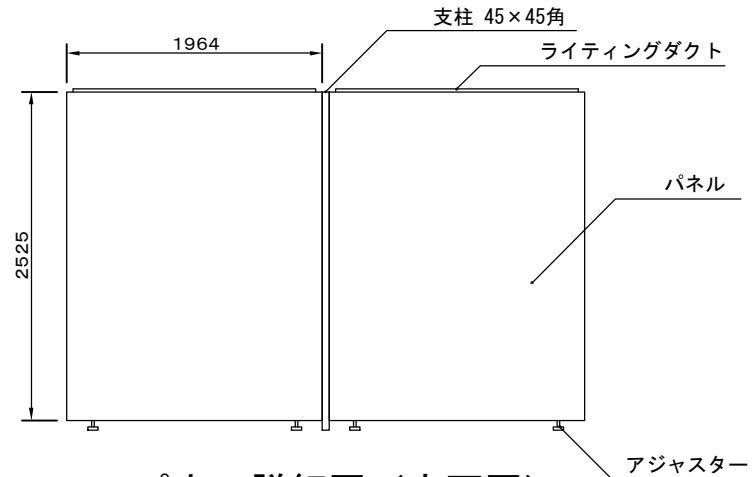
パネル詳細図 (立面図)
